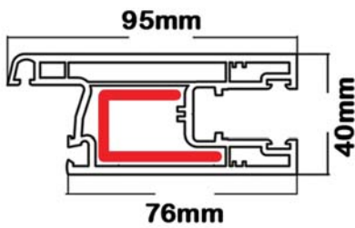
Sliding door sash Profile
