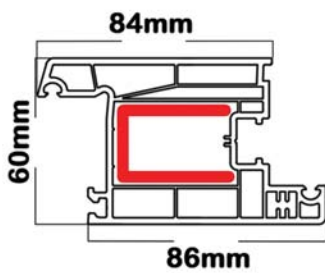
Door Sash profile
